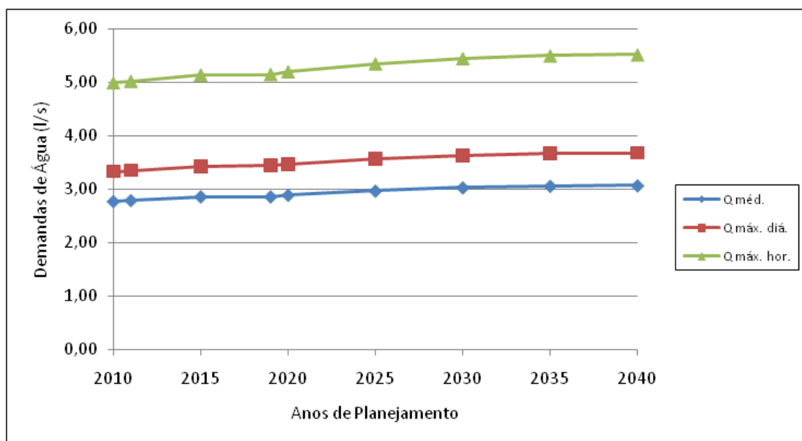
Gráfico 2.5 – Evolução das Demandas/Vazões Disponibilizadas para Distribuição – Distrito dos Cocais
