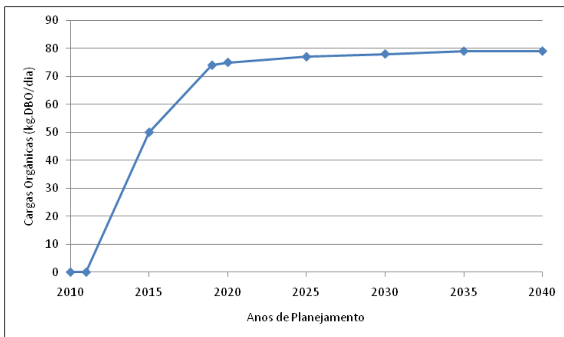
Gráfico 2.12 – Evolução das Cargas Orgânicas Diárias – Distrito dos Cocais
