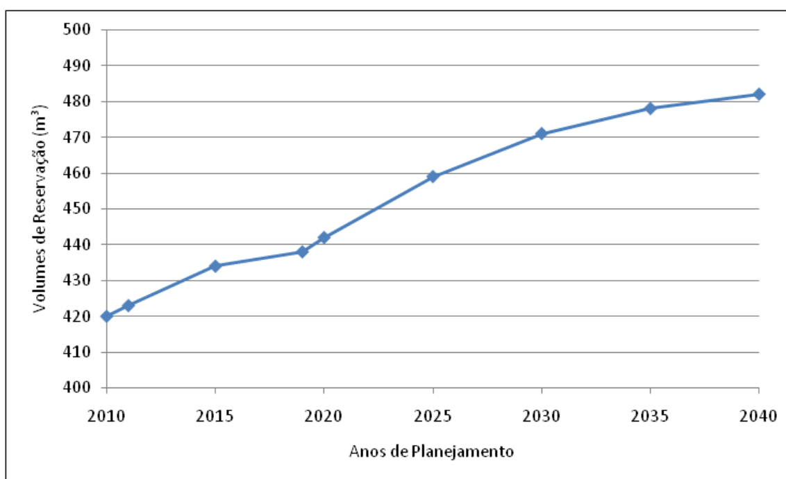
Gráfico 2.4 – Evolução dos Volumes de Reservação Necessários – Distrito Sede
