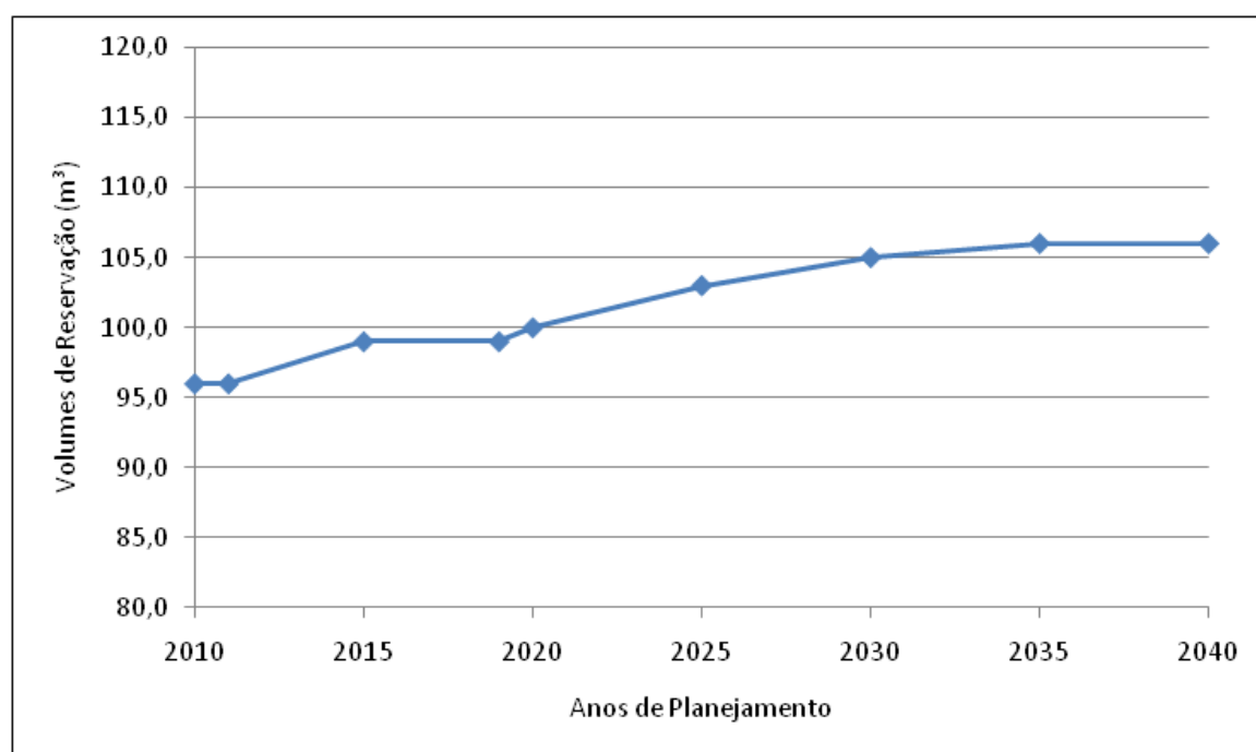
Gráfico 2.6 – Evolução dos Volumes de Reservação Necessários – Distrito dos Cocais
