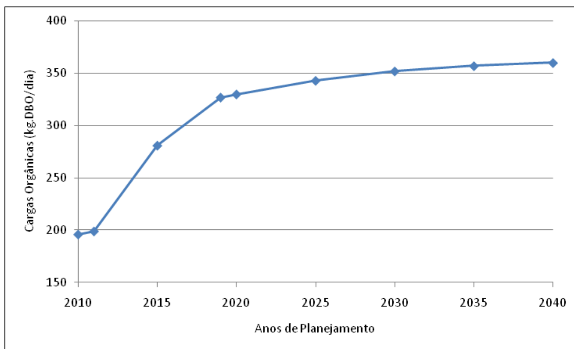
Gráfico 2.10 – Evolução das Cargas Orgânicas Diárias – Distrito Sede
