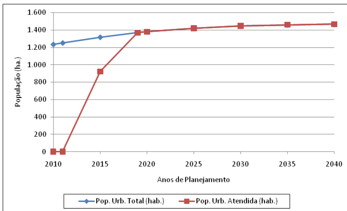
Gráfico 2.8 – População Urbana Total X População Esgotada – Distrito dos Cocais
