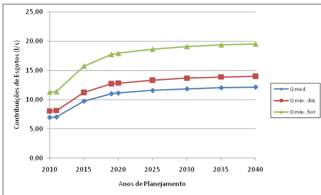
Gráfico 2.9 – Evolução das Contribuições de Esgotos – Distrito Sede
