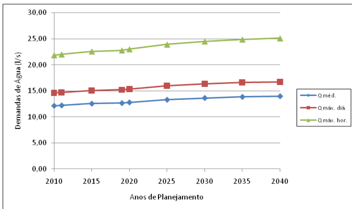
Gráfico 2.3 – Evolução das Demandas/Vazões Disponibilizadas para Distribuição – Distrito Sede
