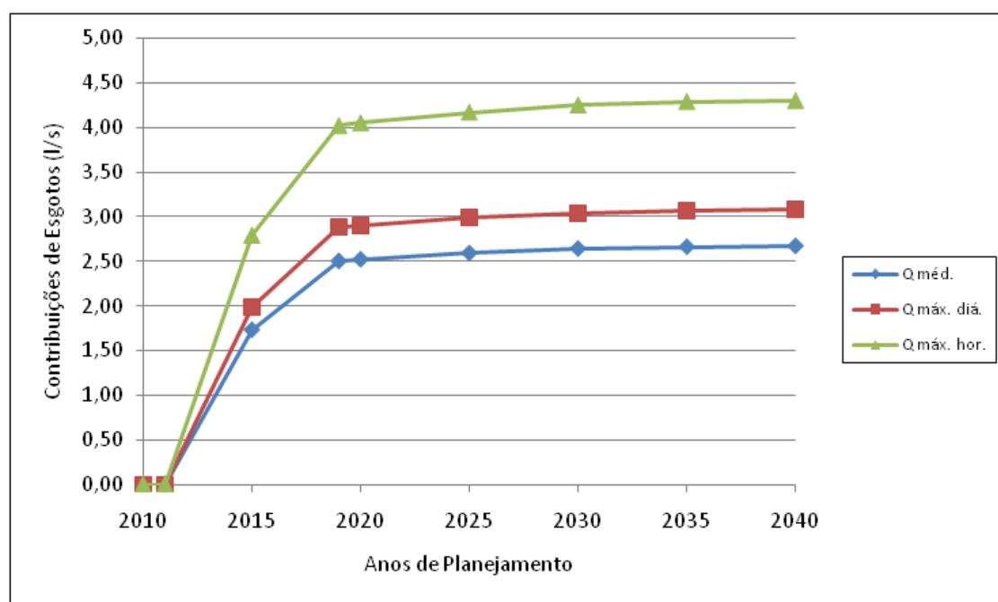
Gráfico 2.11 – Evolução das Contribuições de Esgotos – Distrito dos Cocais
