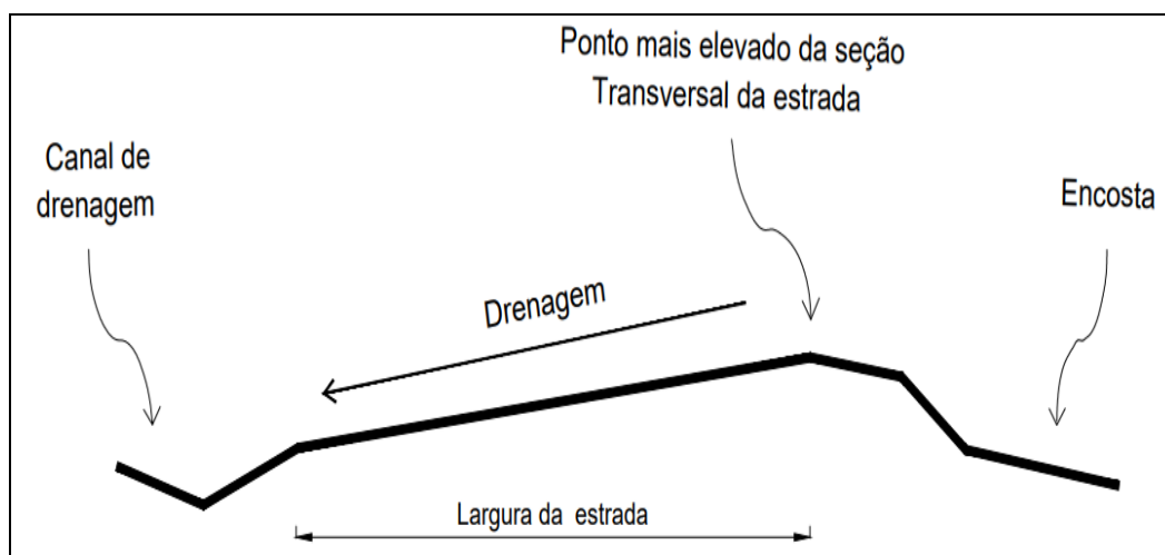
Figura 21 - Perfil Transversal de uma Estrada com Superelevação.
