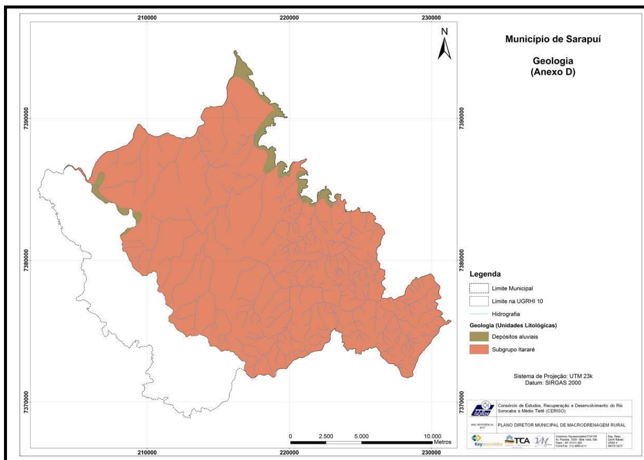
Figura 9 - Geologia de Sarapuí.
