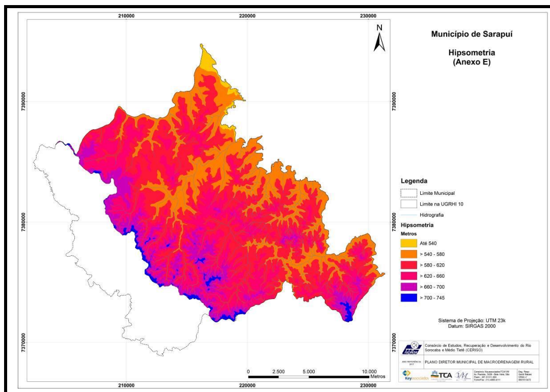
Figura 11 - Hipsometria de Sarapuí.
