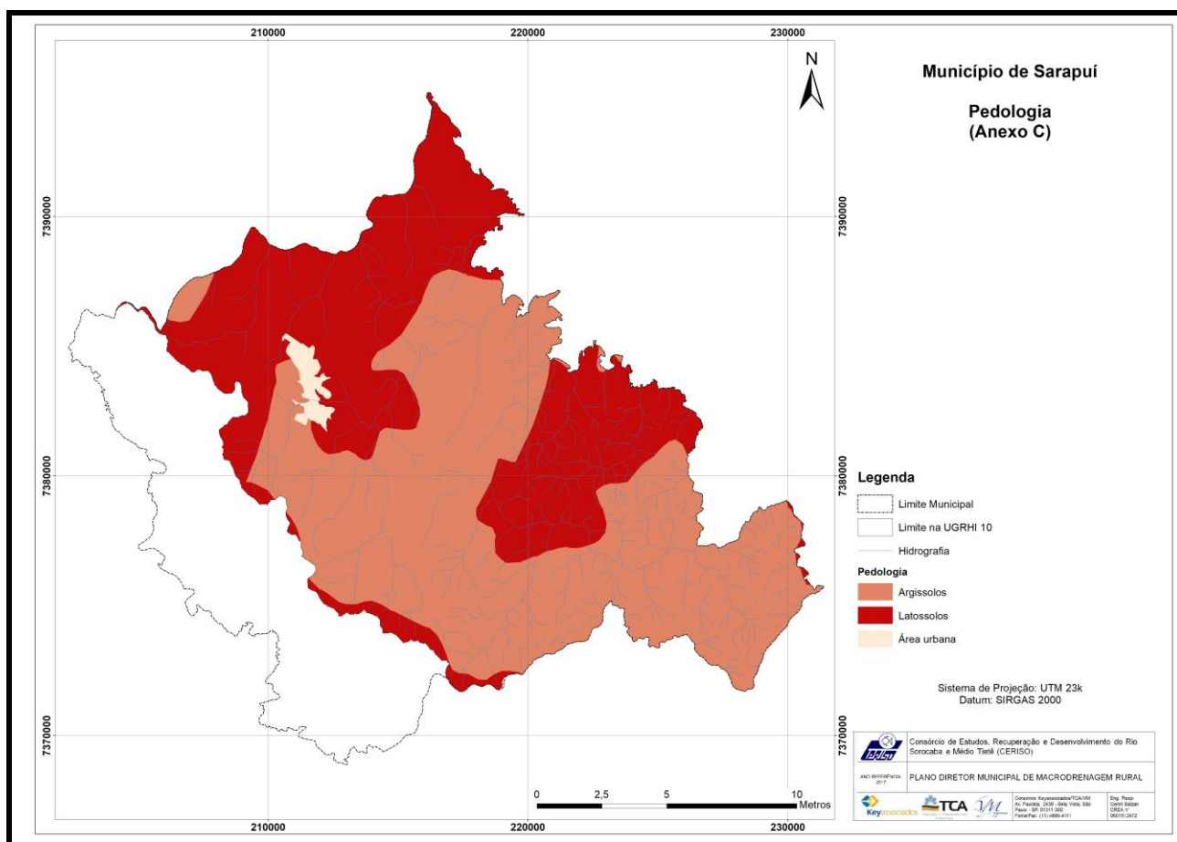
Figura 8 - Pedologia de Sarapuí.
