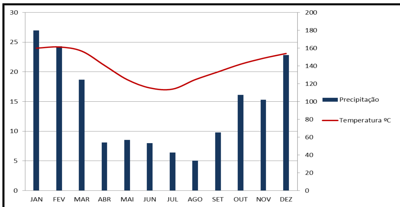
Figura 3 – Precipitação média e temperatura média para Sarapuí.
