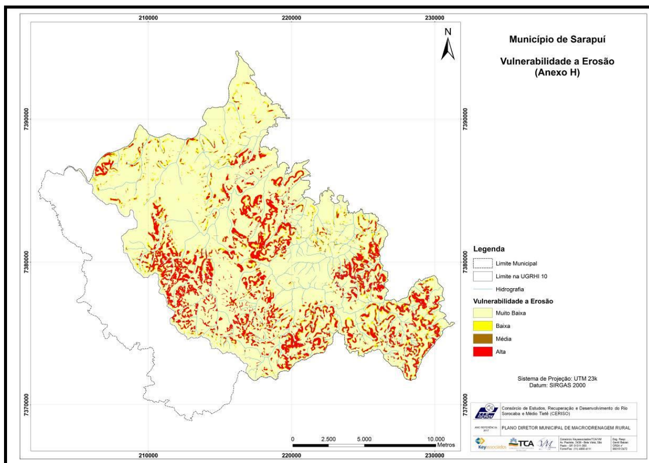
Figura 14 - Vulnerabilidade à Erosão de Sarapuí.
