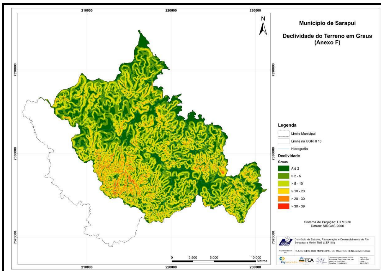
Figura 12 - Declividade do terreno em graus de Sarapuí.
