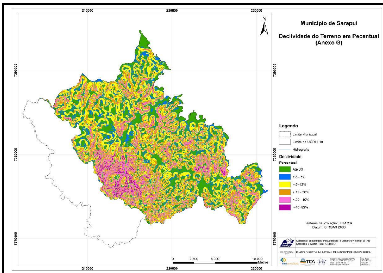
Figura 13 - Declividade do terreno em percentual de Sarapuí.
