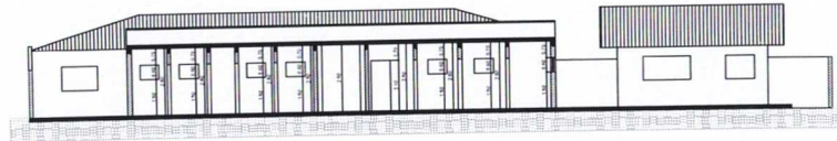
CORTE B-B ESC. 1/100
