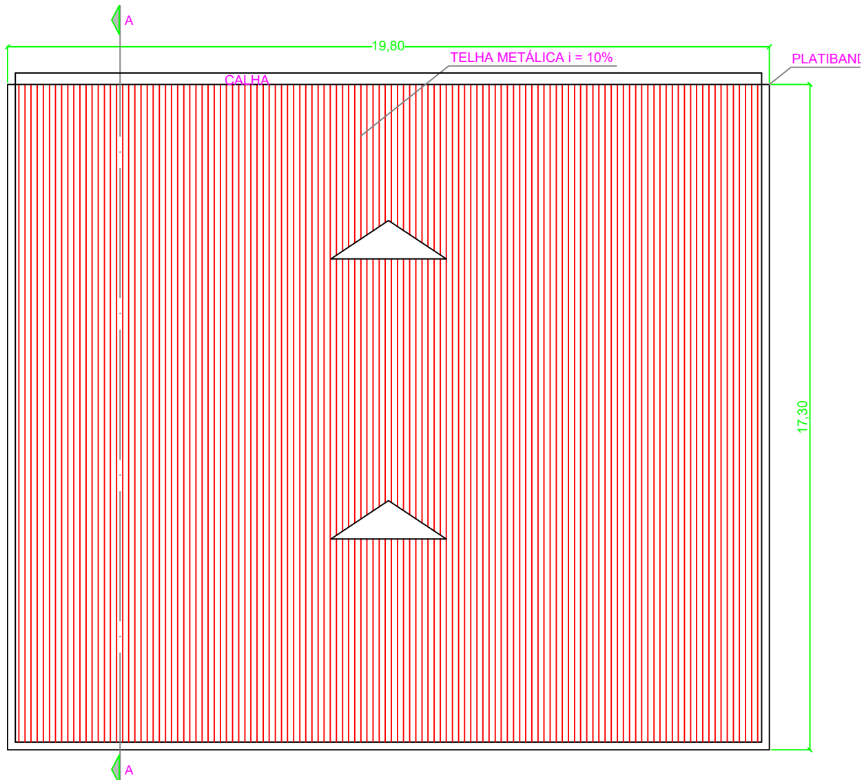
PLANTA COBERTURA ESCALA: 1/125
